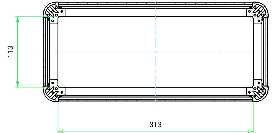
C-C (1 : 3.5)
