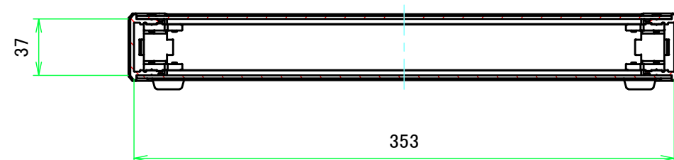
B-B (1 : 3.5)
